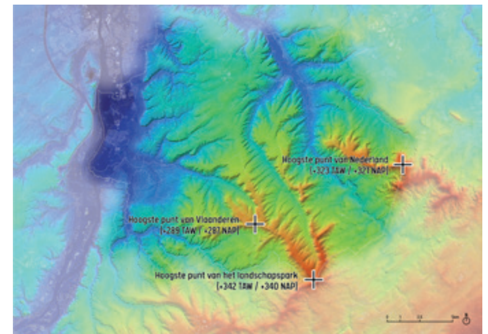
Fig. 1.10- De hoogste punten in het Bocageland
