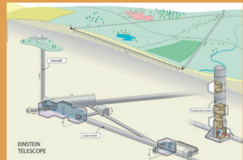
Fig. 1.16- Schets van de ondergrondse detectortunnels van de Einstein Telescoop (200-300m diep) met op elk punt van de driehoek een bovengrondse toren (©T. Balder/Nikhef)
